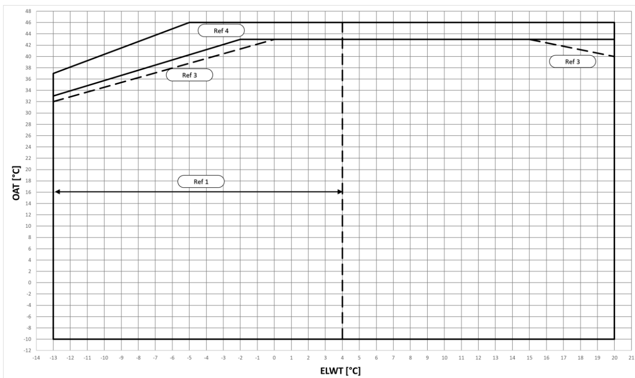
Fig.1– Kufijtë e funksionimit të modalitetit të ftohjes EWYTx5B-S
