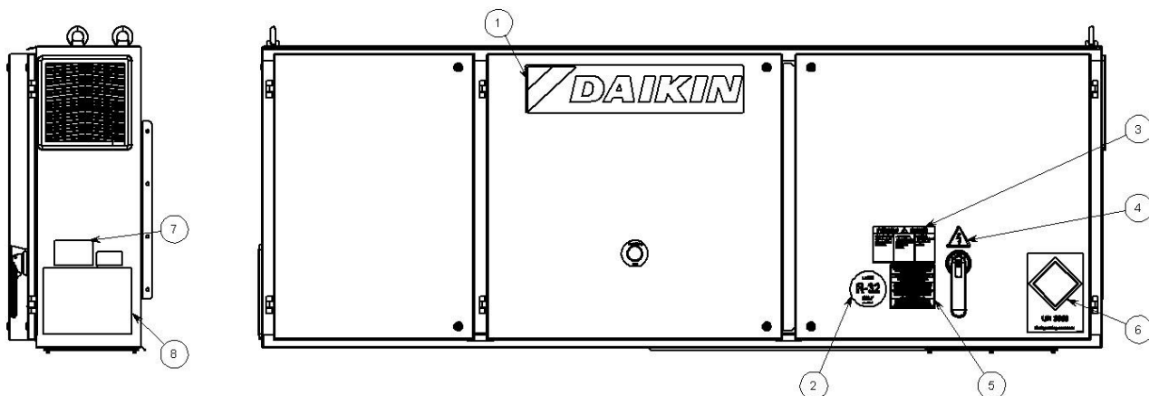
Fik.23– Përshkrimi i etiketave të aplikuara në panelin elektrik EWYTxx0B
