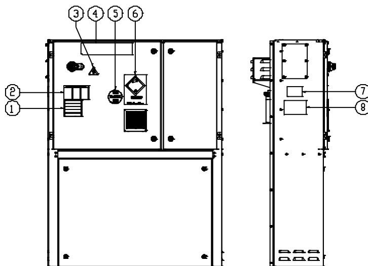
Fik.22– Përshkrimi i etiketave të aplikuara në panelin elektrik EWYTxx5B
