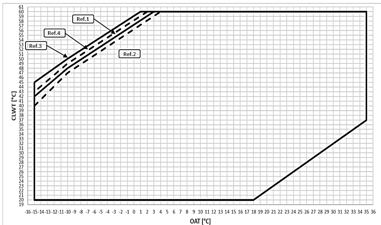
Fik.8– EWYT–BX – OP.204 Kufijtë e funksionimit të modalitetit të ngrohjes
