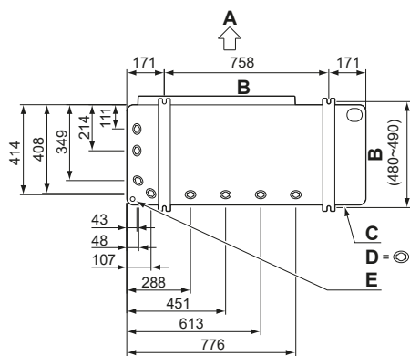
Vrimat e kullimit (dimensionet në mm)
