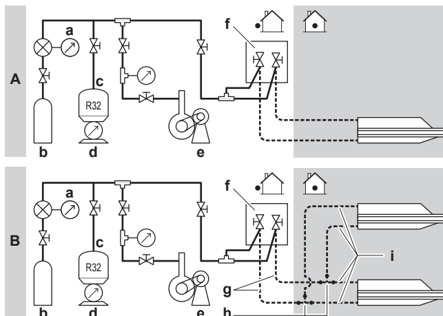
A Instalimi në rastin e çiftit B Instalimi në rastin e dyshes
