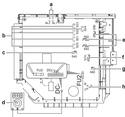
a AL1, AL2 - lidhësi i telit të valvulit solenoid*
