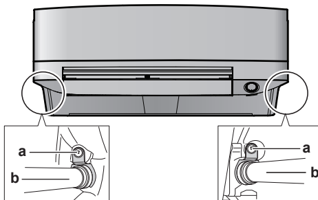
a Vidha e fiksimit të izolimit b Zorra e kullimit
