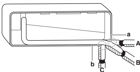
A Tubacioni i krahut të majtë B Tubacioni prapa majtas C Tubacioni fundor majtas a Hiqni kapakun e portës së tubit këtu për tubacionin e krahut të majtë b Hiqni kapakun e portës së tubit këtu për tubacionin e krahut të majtë në fund
